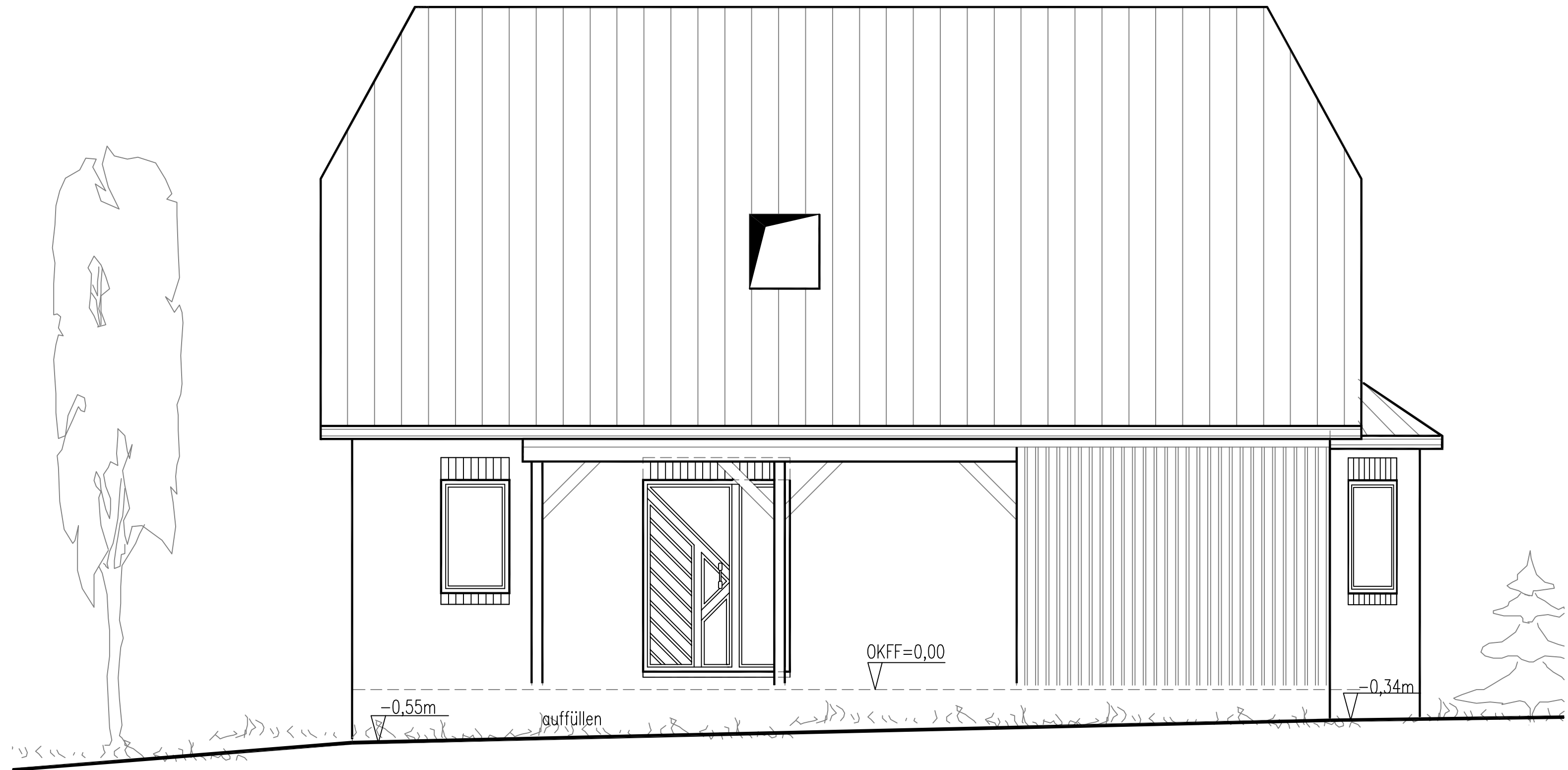
Nordwestansicht
